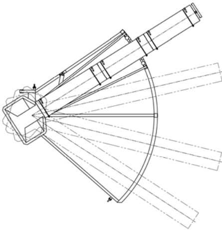
Convoyeur à vis sans fin 4 positions
