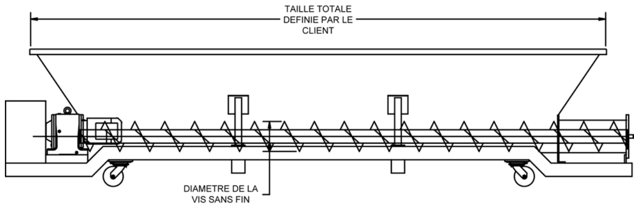
Convoyeur à vis sans fin horizontal
