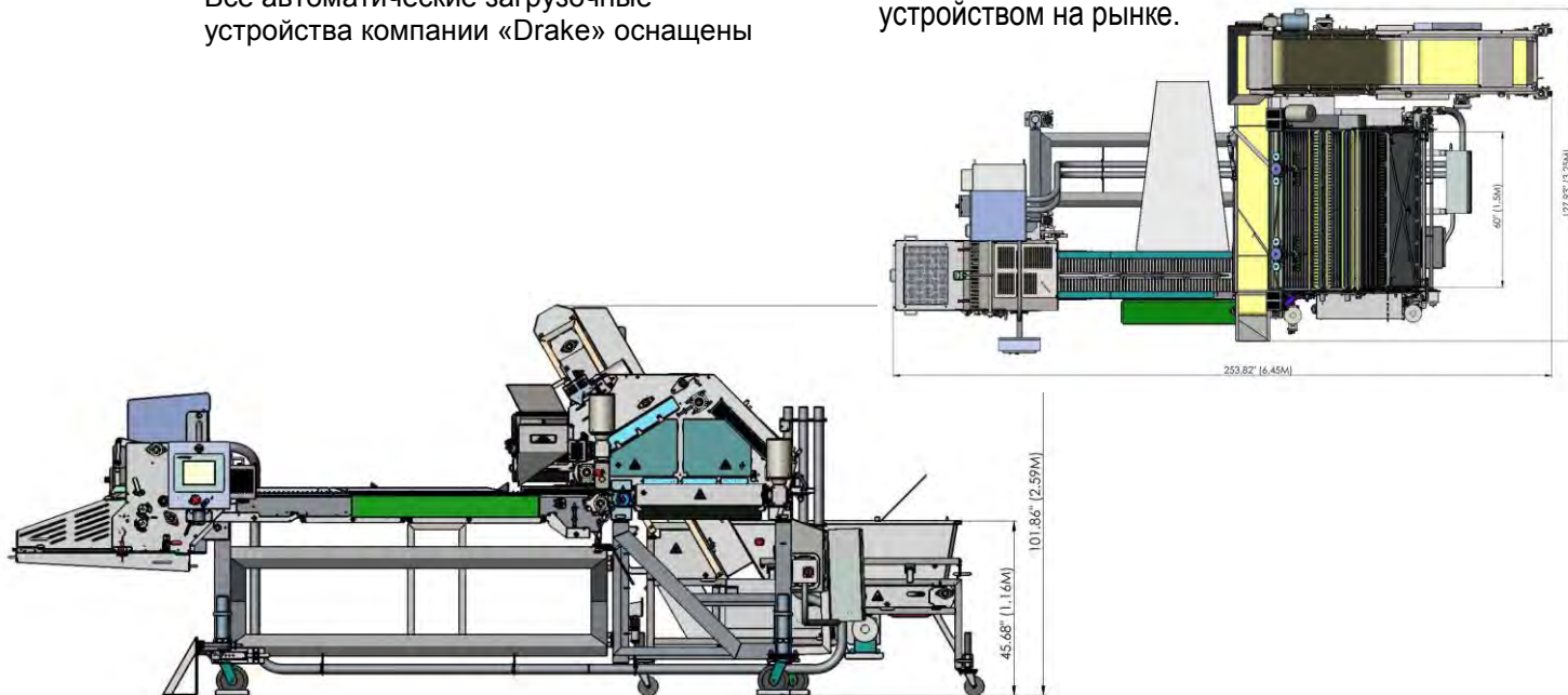
Технические характеристики загрузочного устройства модели CS-1800 компании «Drake»
