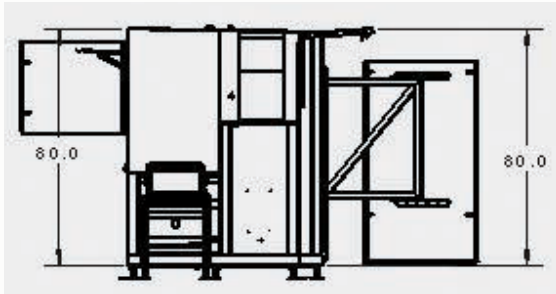
后视图
