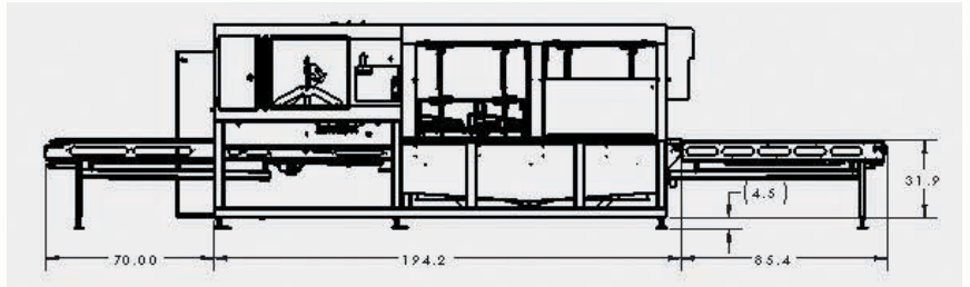
侧视图
